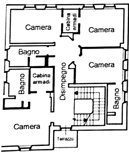
PIANO PRIMO h=3.00m
