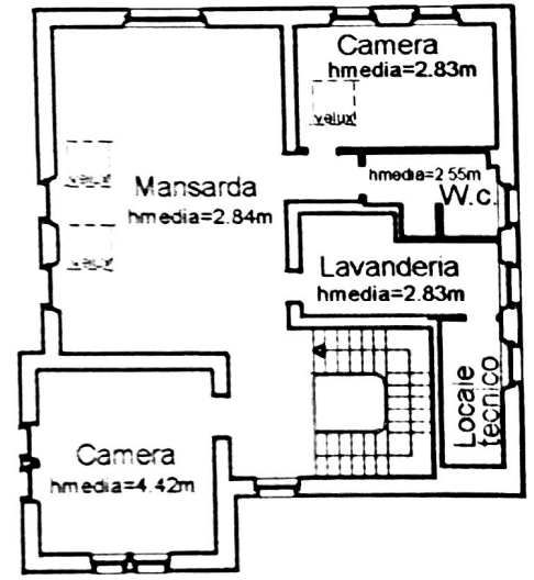
PIANO SOTTOTETTO
